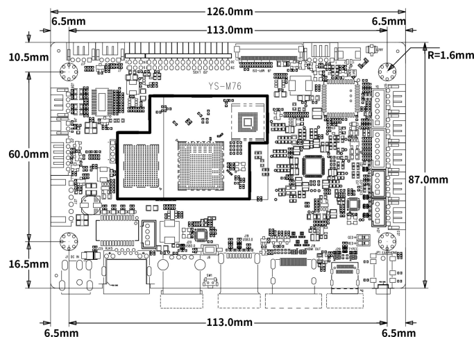
外形尺寸图
