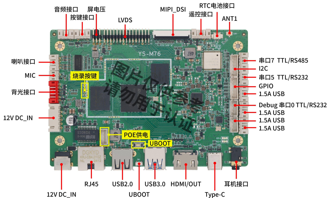
正面接口图
