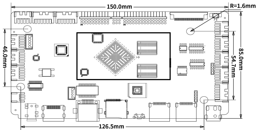
外形尺寸图
