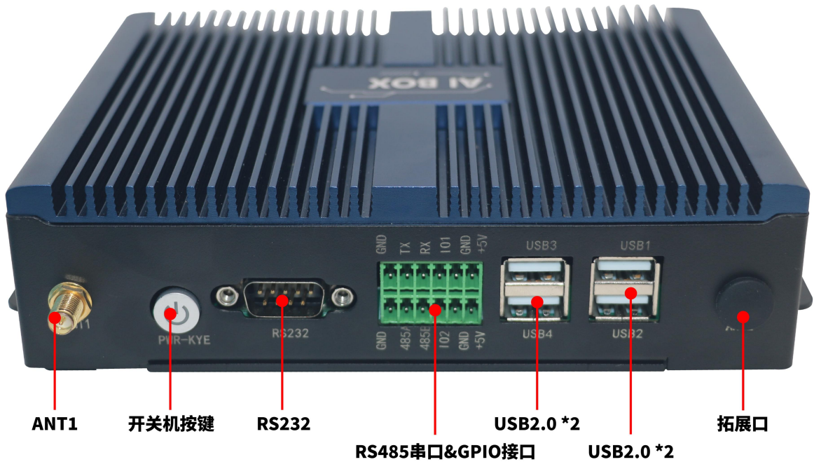
背面图
